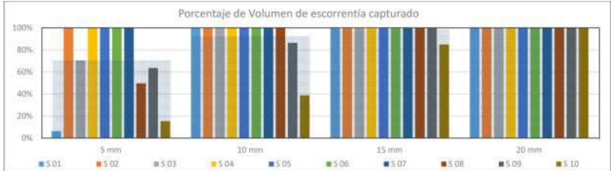
Fig. 5 Porcentajes de los volúmenes de escorrentía capturados para cada suceso (S01 a S10) en función de los mm de precipitación o “WQv”.
