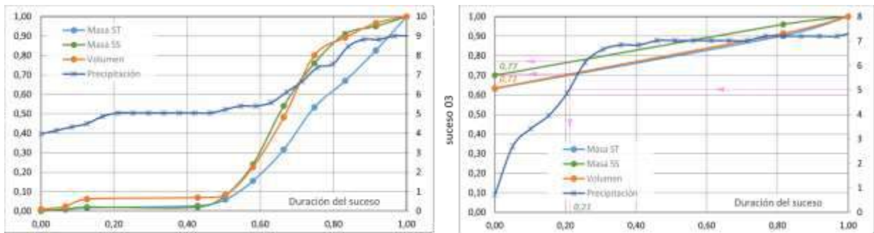
Fig. 3 Volumen, SS, ST [normalizados] y precipitación [mm] acumulados en el suceso 1 y suceso 3.
