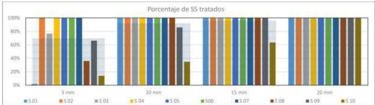
Fig. 6 Porcentajes de masa de SS tratada en función de los mm de lluvia capturada en cada suceso y valor medio.
