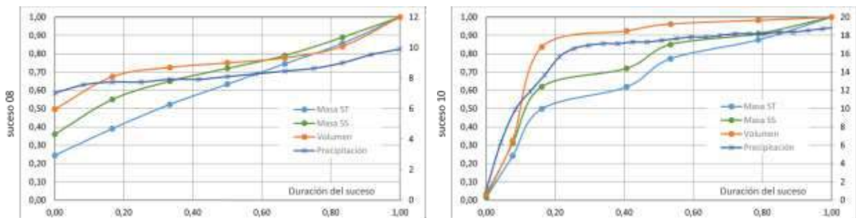
Fig. 4 Volumen, SS, ST [normalizados] y precipitación [mm] acumulados en el suceso 8 y suceso 10.
